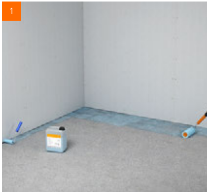
1 Grundierung des Untergrundes mit fermacell™ Tiefengrund
