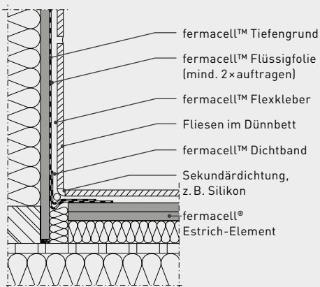
Boden-Wand-Anschluss
